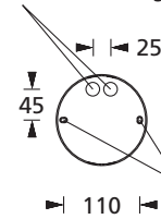
Kabeleinführung
