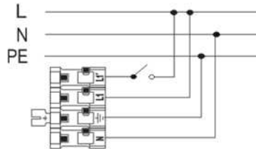
Nr. 2 Dauerschaltung mit externem Schalter
